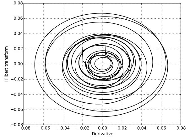
b) PC 1, \tau_x
