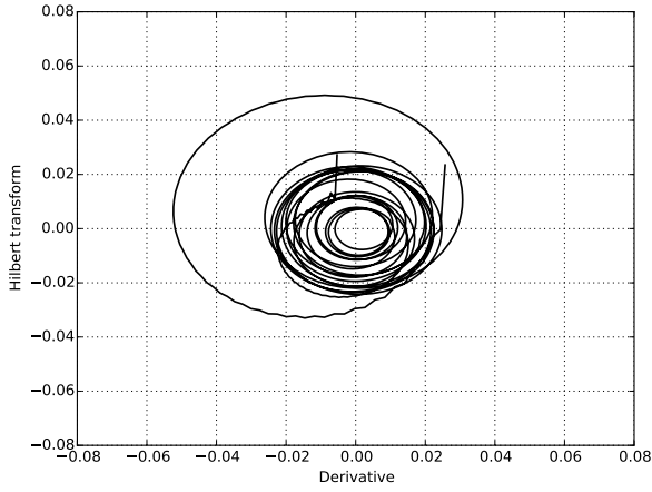
a) KE path length
