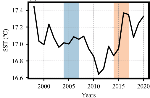
(d) Bohai Sea in China
