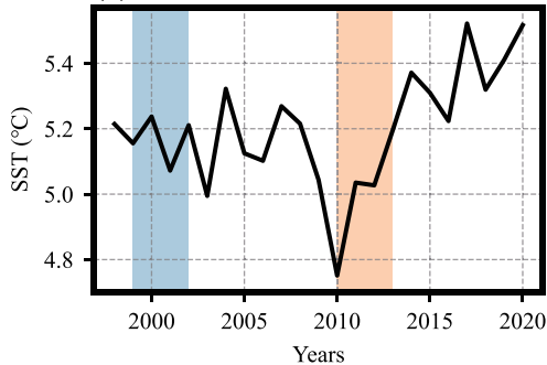
(d) Bohai Sea in China
