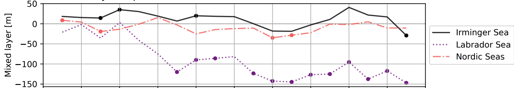
(d) Mixed layer depth
