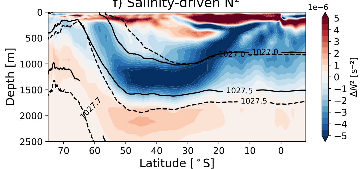
f) Salinity-driven N^2
