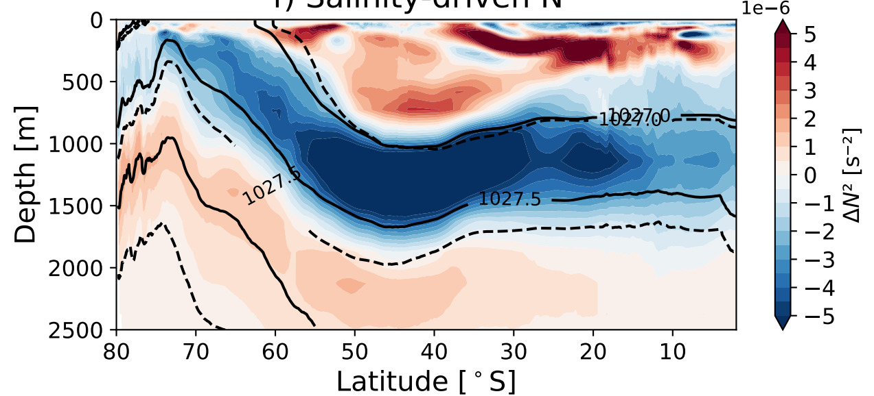
f) Salinity-driven N^2
