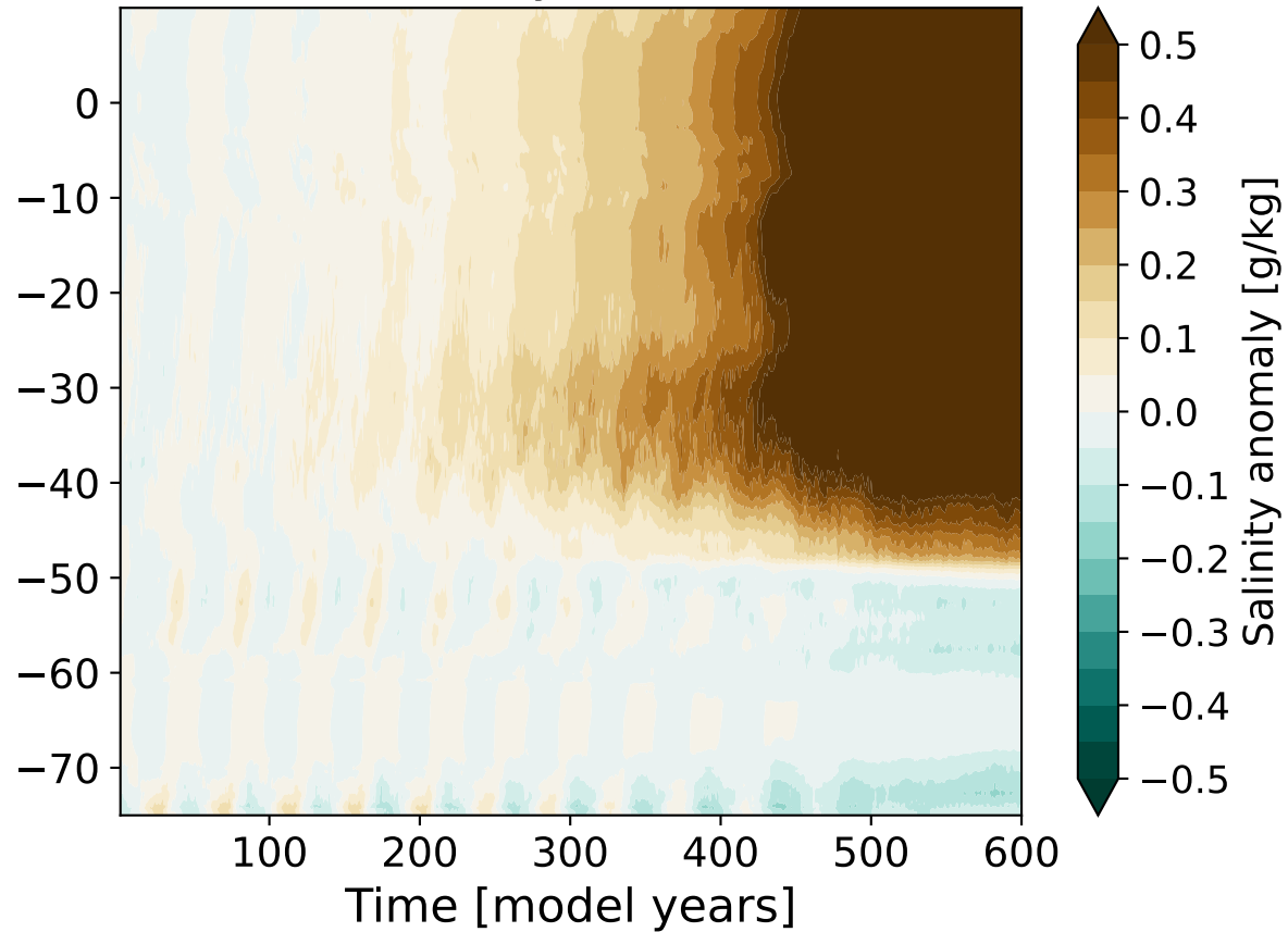
b) Salinity anomalies
