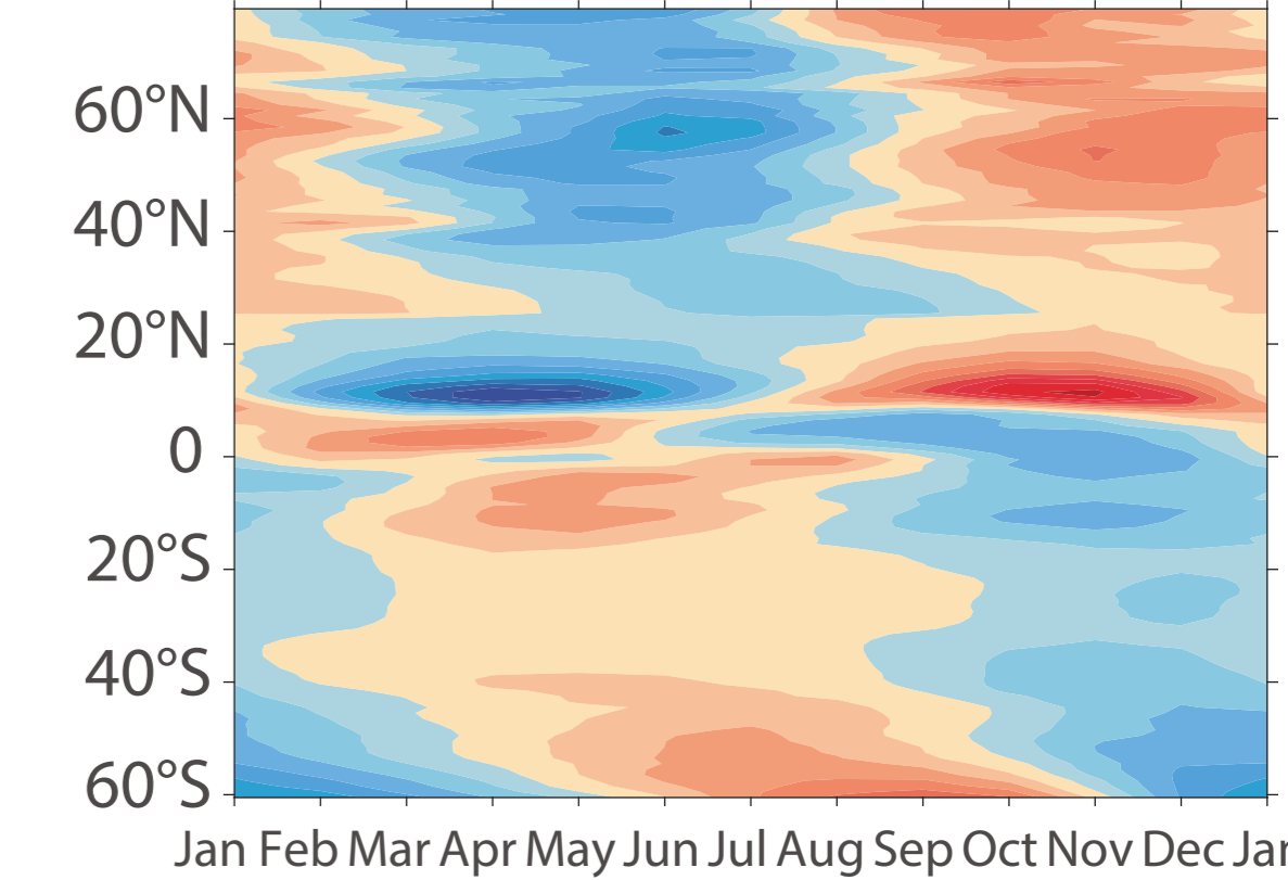
AOU_GOBAL
