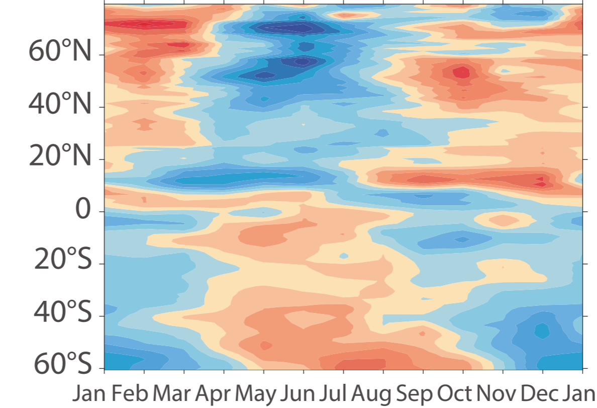
AOU_WOA18
