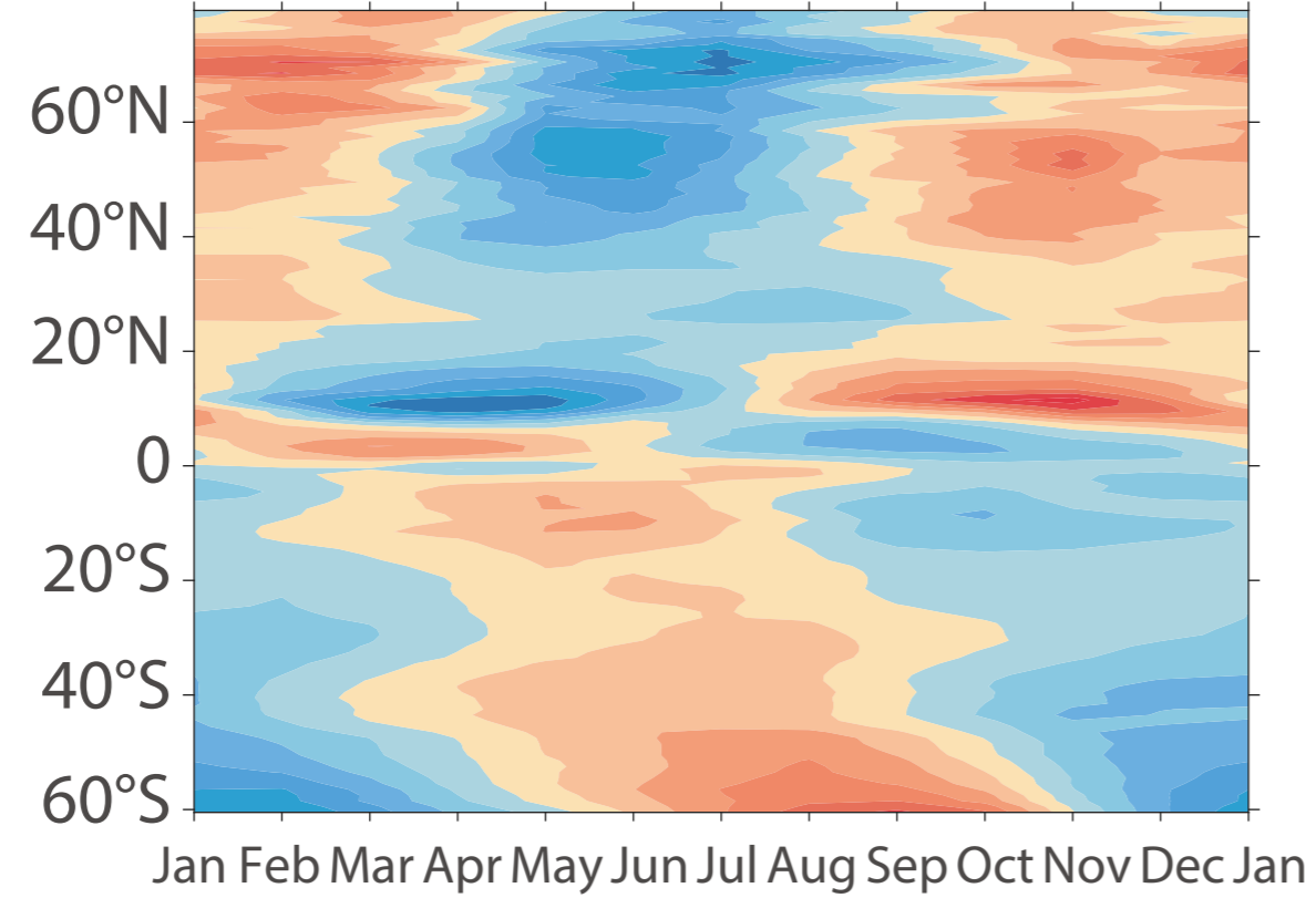
AOU_IAP
