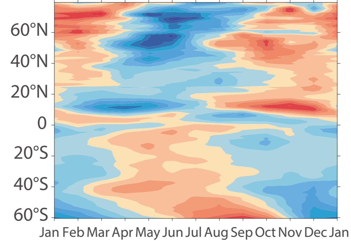
AOU_WOA23
