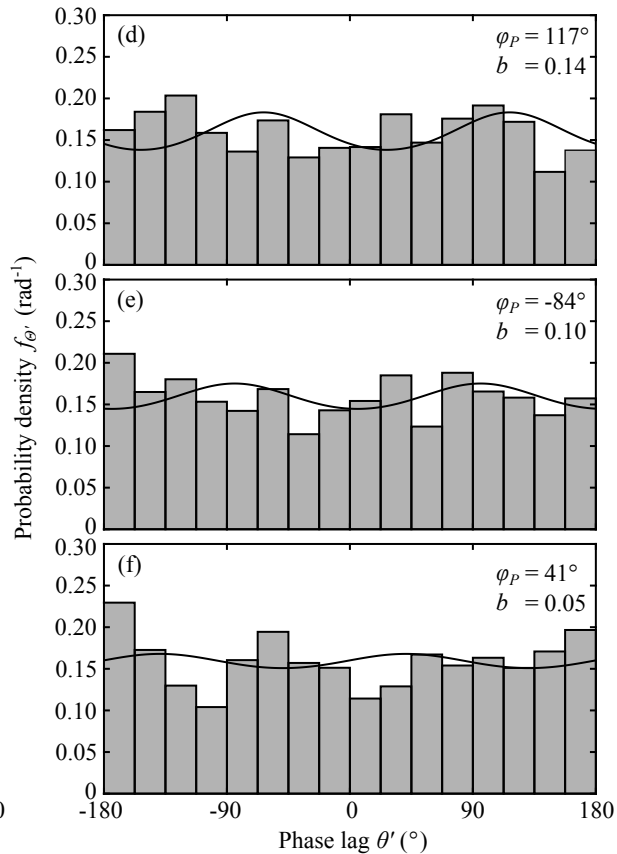
Phase lag
