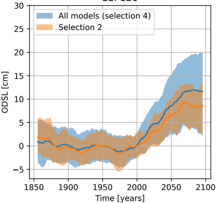
SSP126
