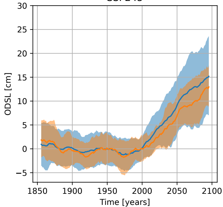
SSP245
