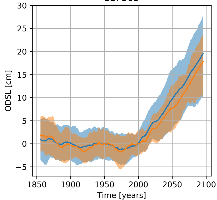
SSP585
