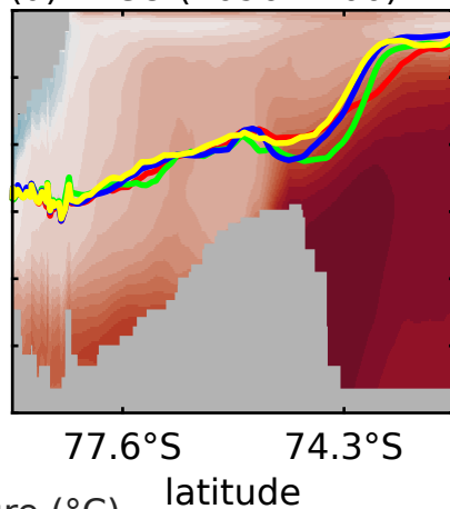
(d) FECO (2096-2100)
