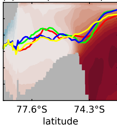
(d) FECO (2096-2100)
