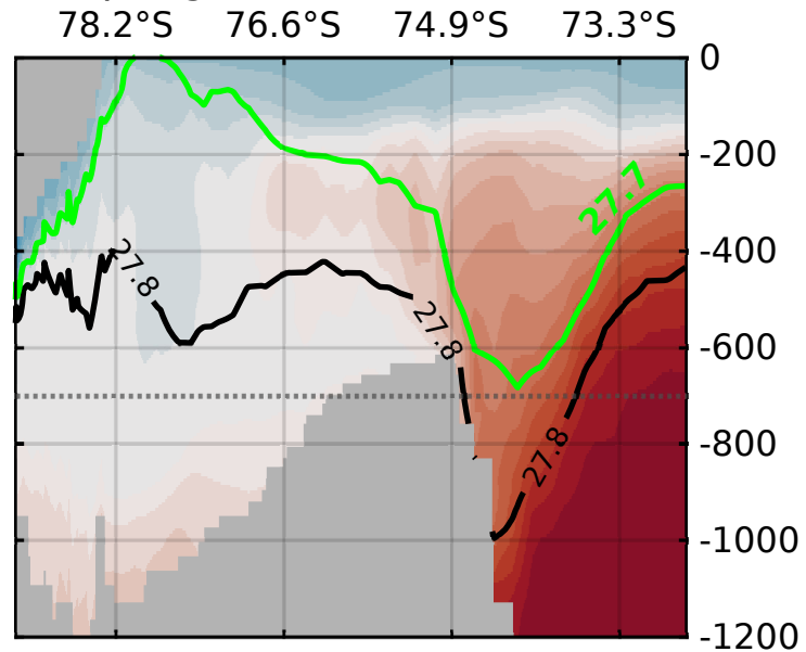
(d) autumn
