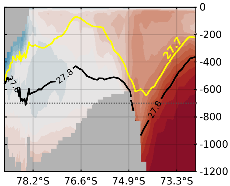
(d) autumn
