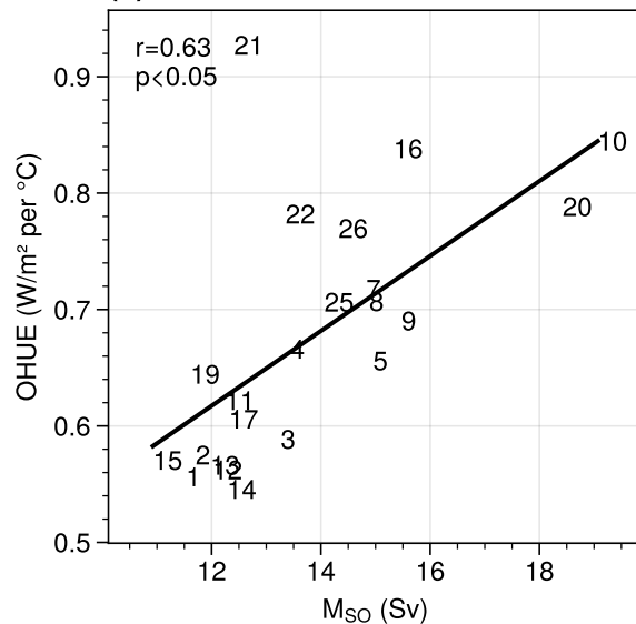
(d) M_{SO} vs. OHUE
