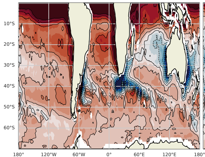
(d) B^{\text{surf}} OAflux raw
