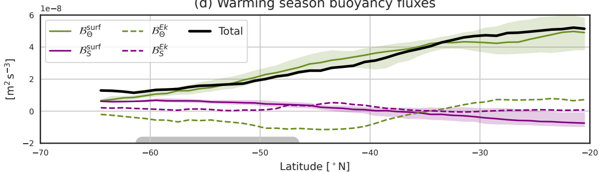
(d) Warming season buoyancy fluxes
