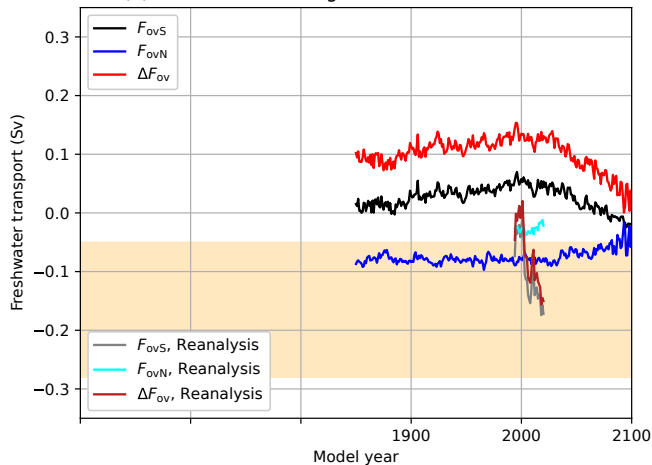
(d) Freshwater convergence, LR-CESM, Hist/RCP8.5
