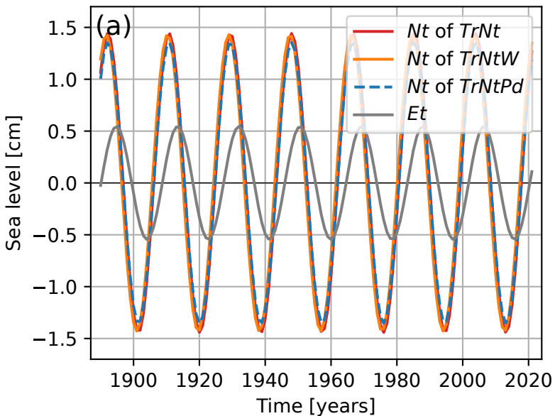
Nodal tide
