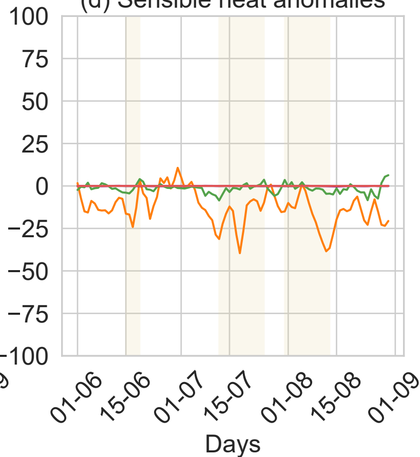
(d) Sensible heat anomalies
