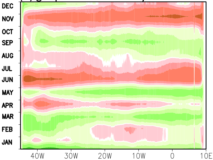
(d) geopotential anomaly : BCM2
