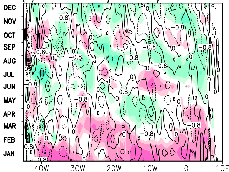
(e) zonal velocity anomaly : BCM3
