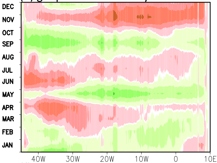
(f) geopotential anomaly : BCM3
