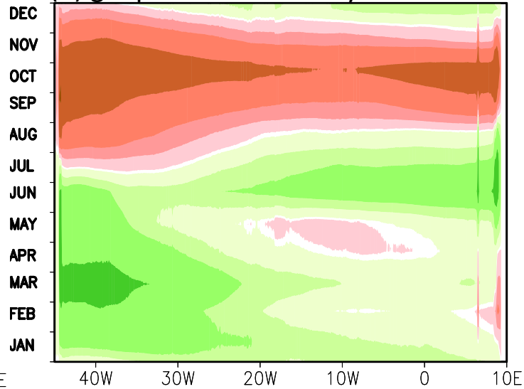
(d) geopotential anomaly : BCM2
