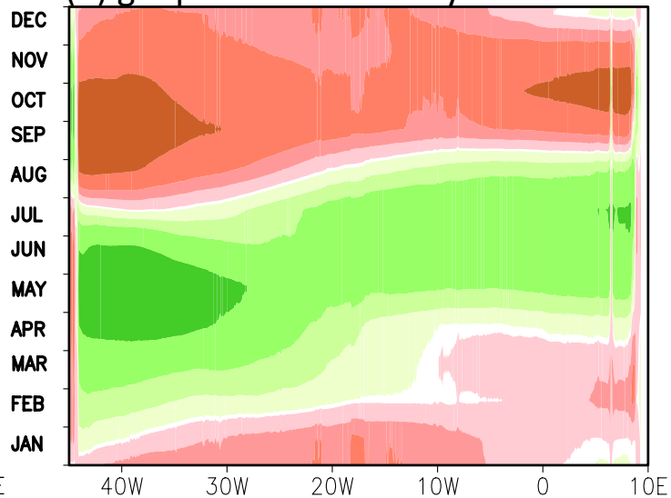
(f) geopotential anomaly : BCM3
