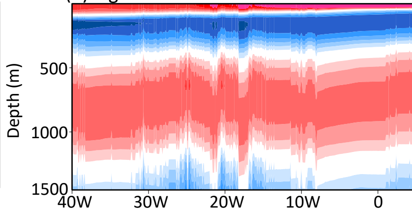
(d) Eigenfunction: BCM4
