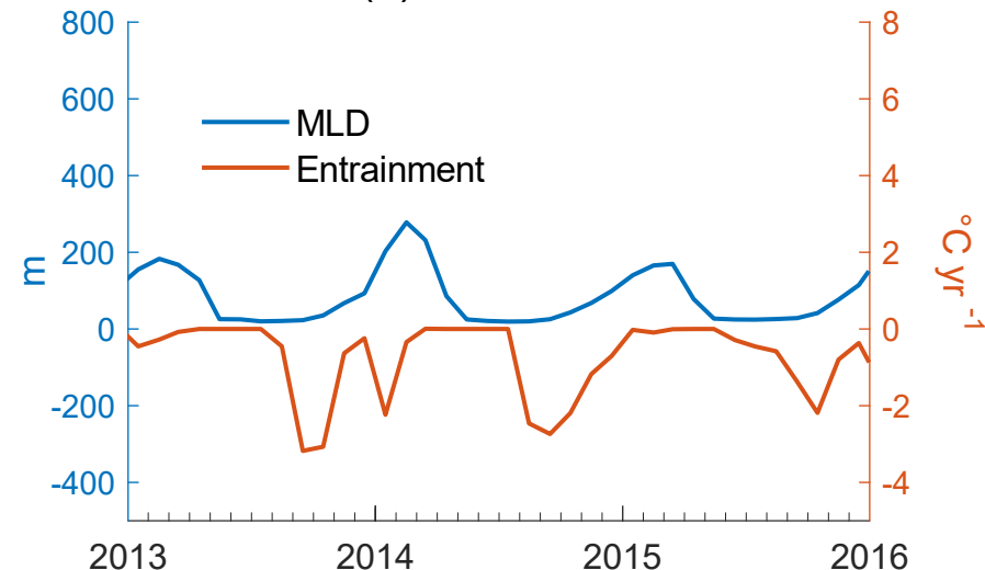
(d) MLD: south
