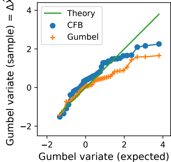
(d) VdBK08 (QQ) plot, Observations
