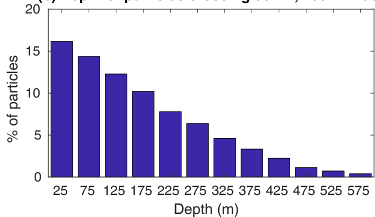
(d) Depth of particles crossing 30° W, 2010 hindcast
