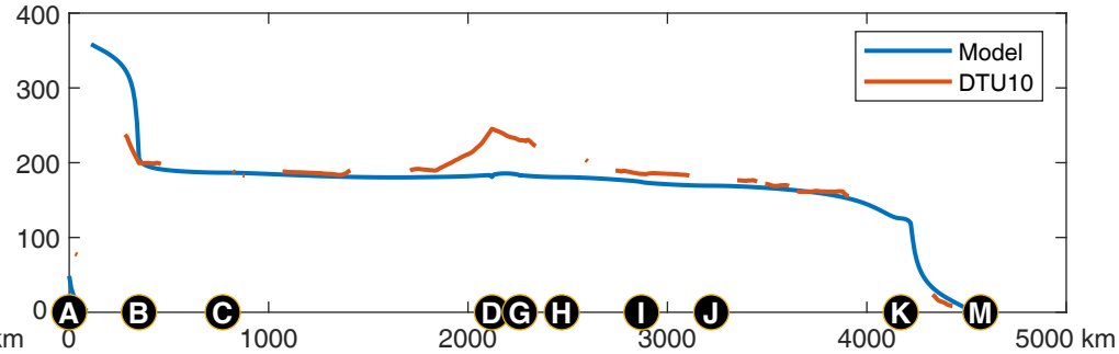
(d) Phase lags (degree) of M_2 tide
