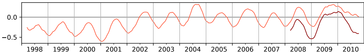
(d) Primary production (free run)
