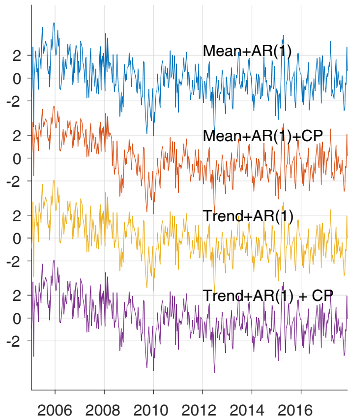
(b) AR(1) plus mean / trend / CP
