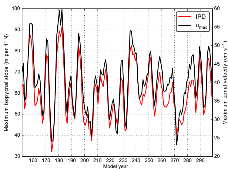
(d) Maximum isopycnal slope and zonal velocity
