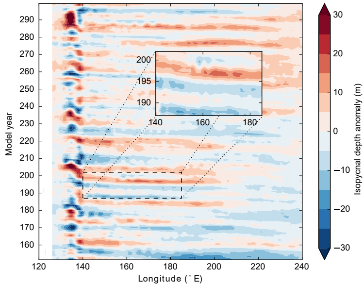
(b) IPD Hovmöller
