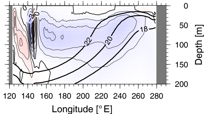
(b) W reg. Nino3, OLD
