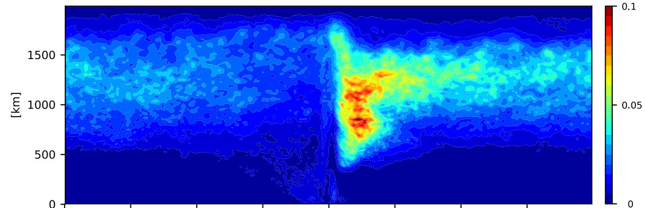
(f) \langle w'b' \rangle_{(0-500m)} [10^{-8}m^2s^{-3}] - R+R
