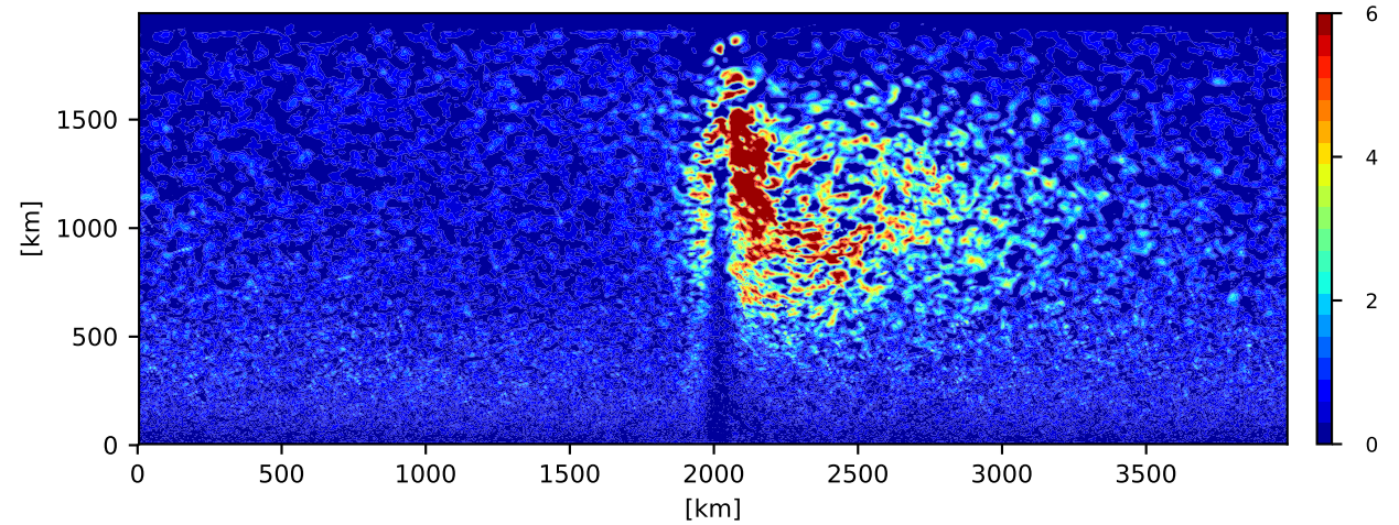
(c) \langle w'b' \rangle_{(0-500m)} [10^{-8}m^2s^{-3}] - R+F
