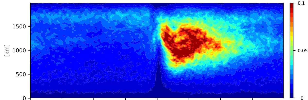
(c) \langle w'b' \rangle_{(0-500m)} [10^{-8}m^2s^{-3}] - R+F
