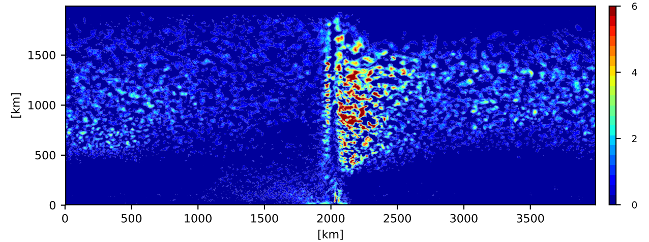
(f) \langle w'b' \rangle_{(0-500m)} [10^{-8}m^2s^{-3}] - R+R
