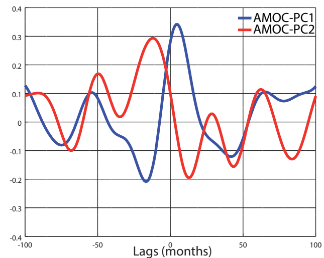
(d) Corre(AMOC, PCs-WB f800m) GC2
