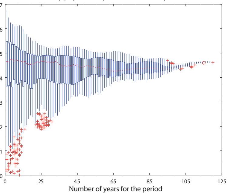
(e) r(PC1 WB, AMOC 900m Nf)
