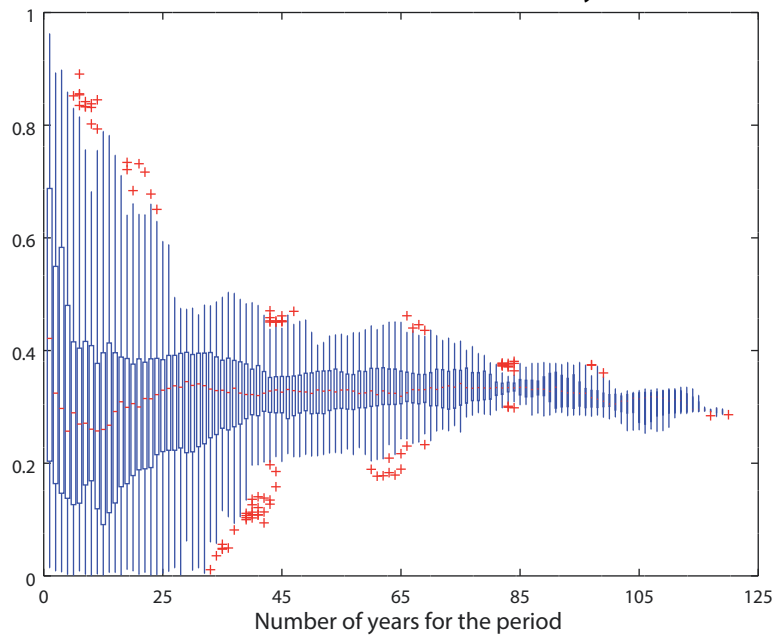
(f) r(PC2 WB, AMOC 900m) F>2yr
