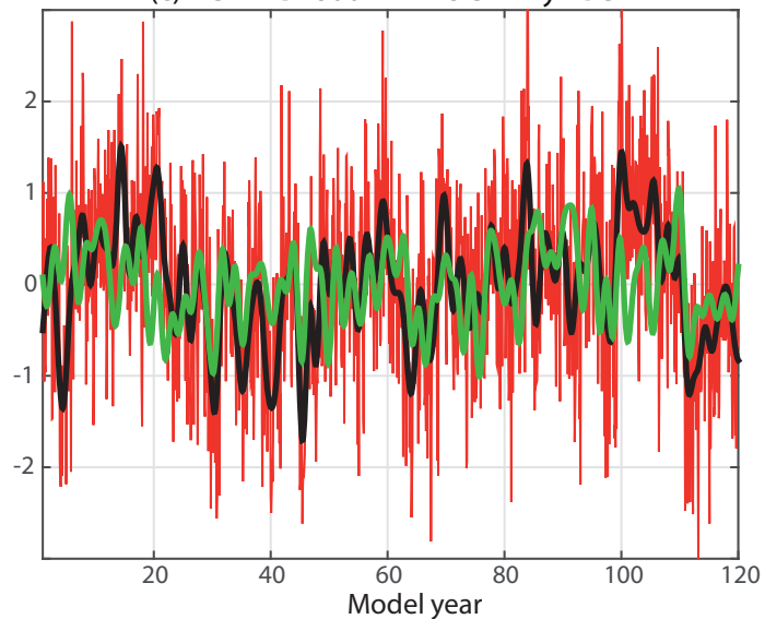
(f) r(PC2 WB, AMOC 900m) F>2yr
