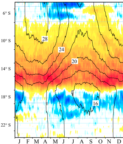
(a) OISST
