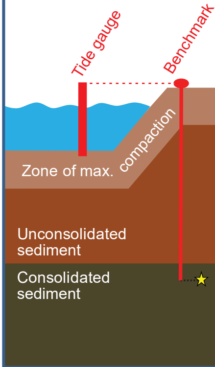
(b) Thin LECZ
