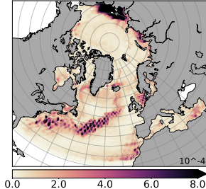
(b) Updated ensemble : spatial localisation only
