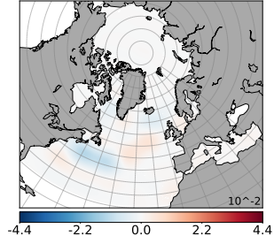
(a) Analysis increment : spatial localisation only
