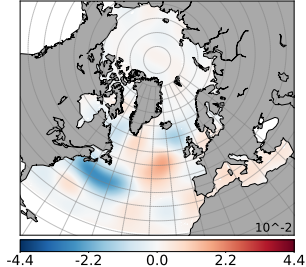
(b) Analysis increment : spectral localisation only
