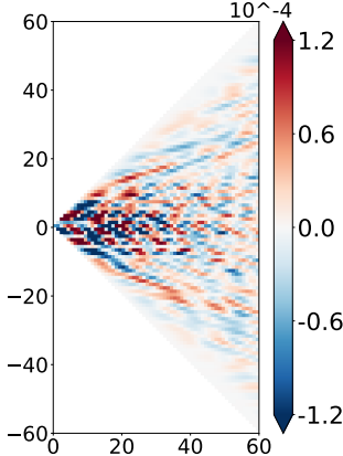
(b) True anomaly
