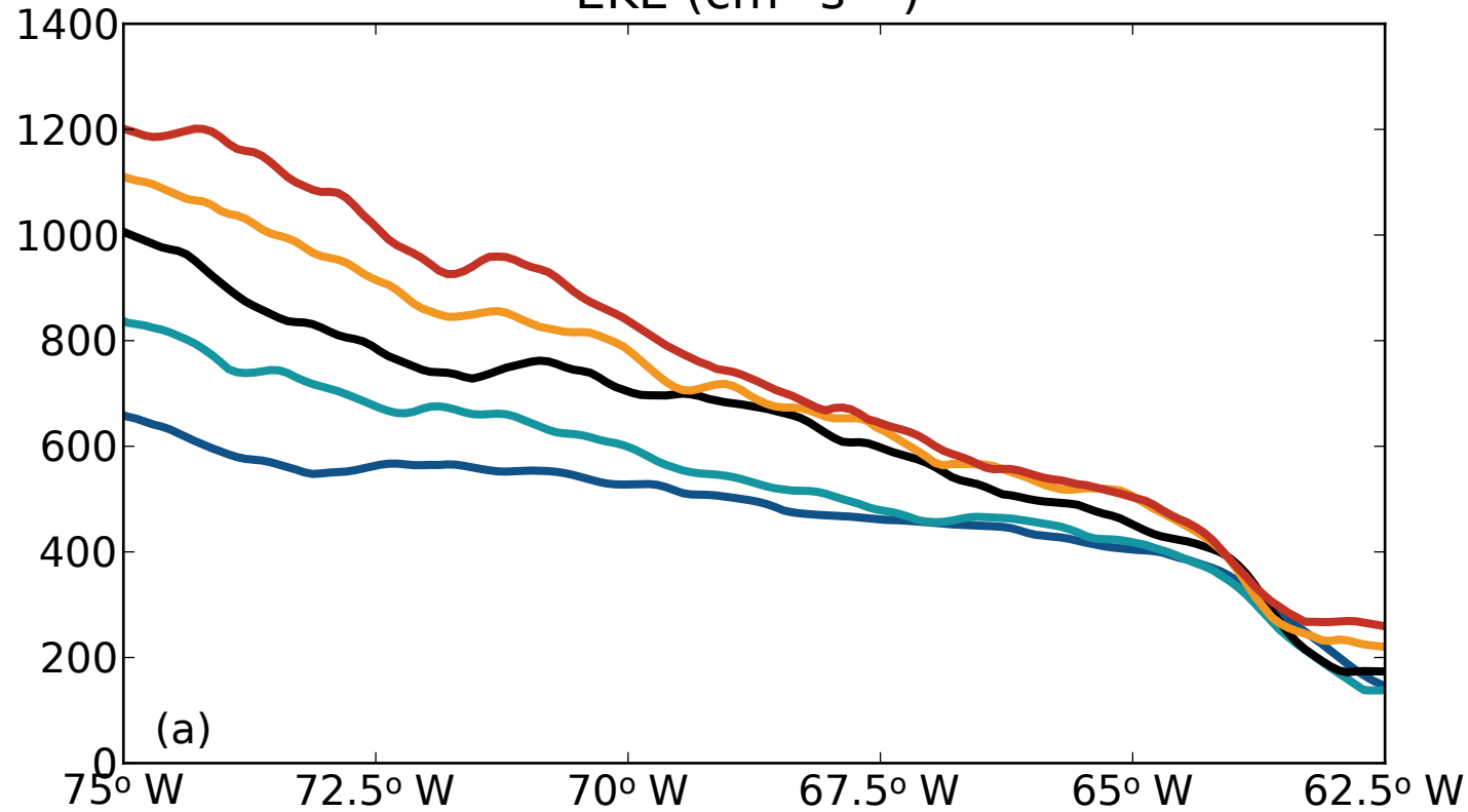
EKE ( \text{cm}^2 \text{s}^{-2} )
