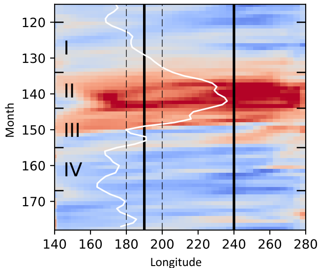
(a) SST anomalies and ONI
